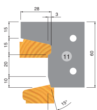
Profil 11 Listello fermavetro / Rejet d'eau
