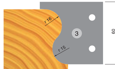
Profil 3 Corrimano / Main courante
