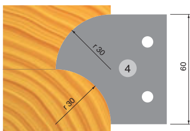
Profil 4 Doppio raggio / Bec de Corbin
