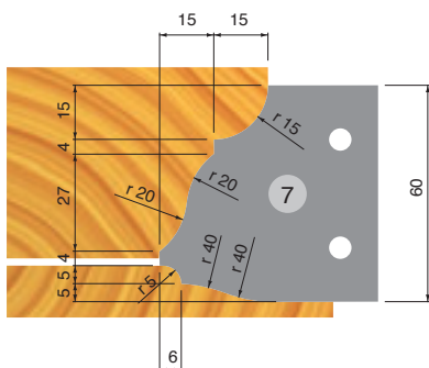
Profil 7 Profilo cornice/piattabanda / Alaise + plate bande
