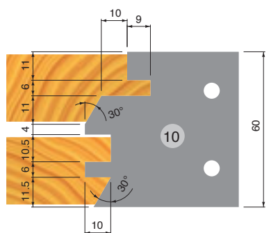
Profil 10 Parchetto / Rainure et Languette
