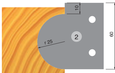
Profil 2 Gola / Congés R25mm
