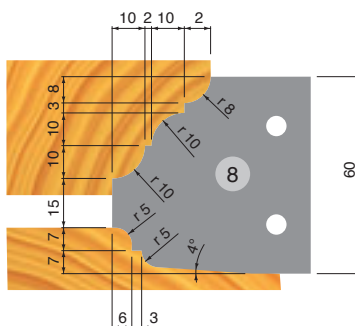
Profil 8 Profilo cornice/piattabanda / Alaise + plate bande
