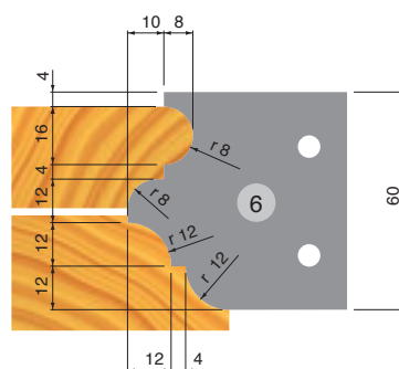
Profil 6 Profili listello A / Multi profil A
