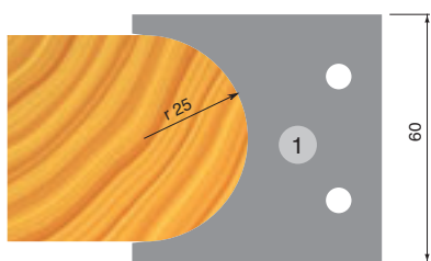
Profil 1 Mezzotondo / 1/2 rond R25mm
