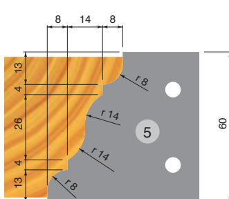
Profil 5 Cornice / Profil cornice
