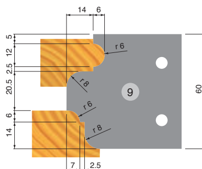
Profil 9 Profili Listello B / Multi profil B
